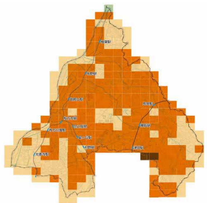
生駒断層帯地震
