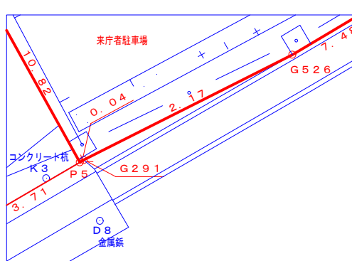
詳細図 B
