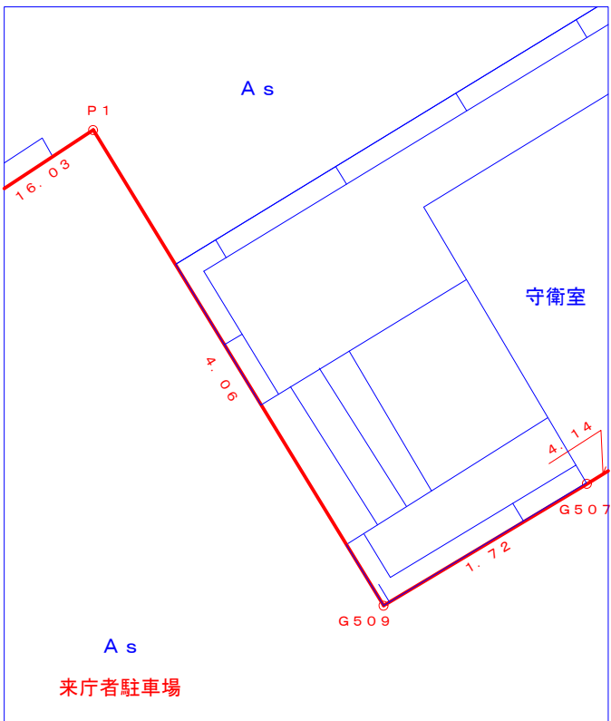
詳細図 A
