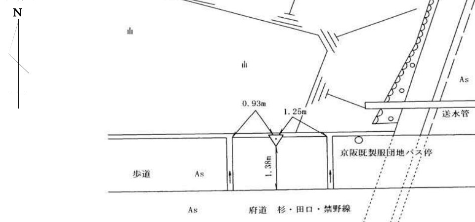
要図
