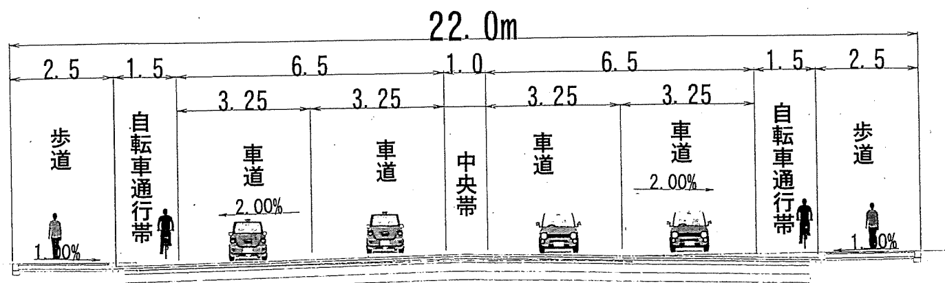
牧野橋以北道路図面 現在の植栽はすべて伐採されます
