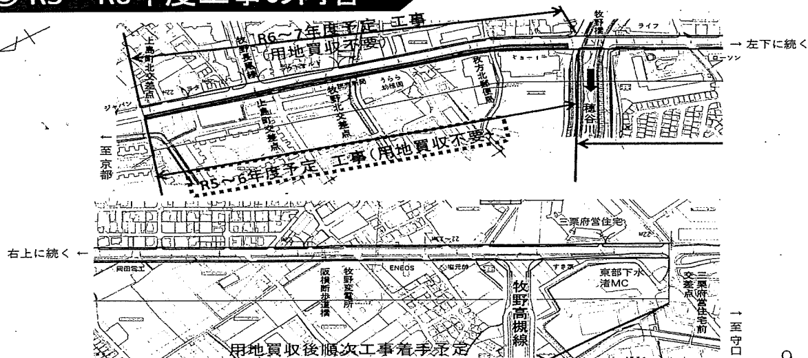
京都守口線 都市計画 平面図
