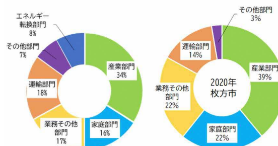
図. 2020年度のCO 2 の部門別構成割合
