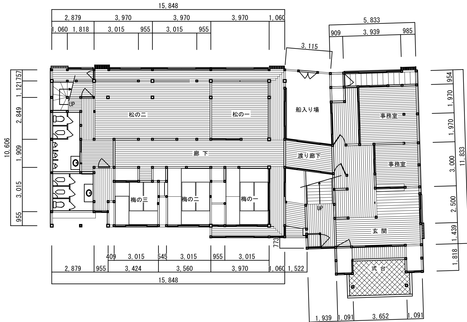
別棟 1階平面図 1/150
