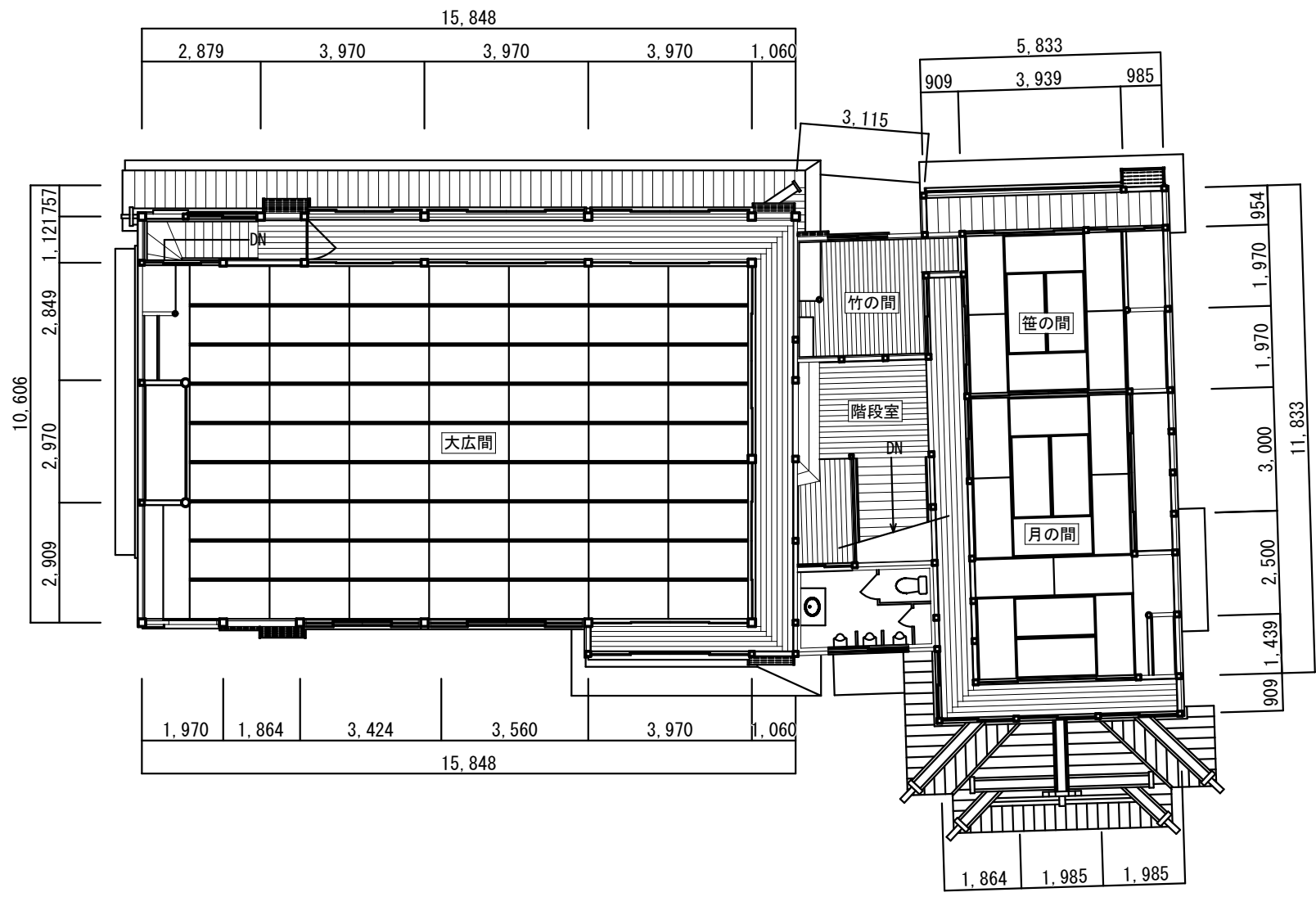
別棟 2階平面図 1/150
