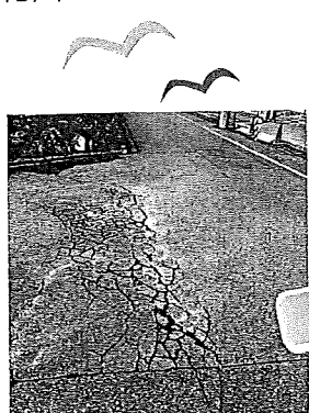
牧野駅前道路補修前
