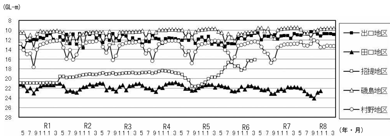
地下水位（静水位）の月平均値の変化
