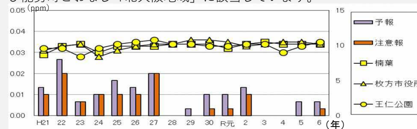
図 光化学オキシダントの推移と光化学スモッグの発令階数
