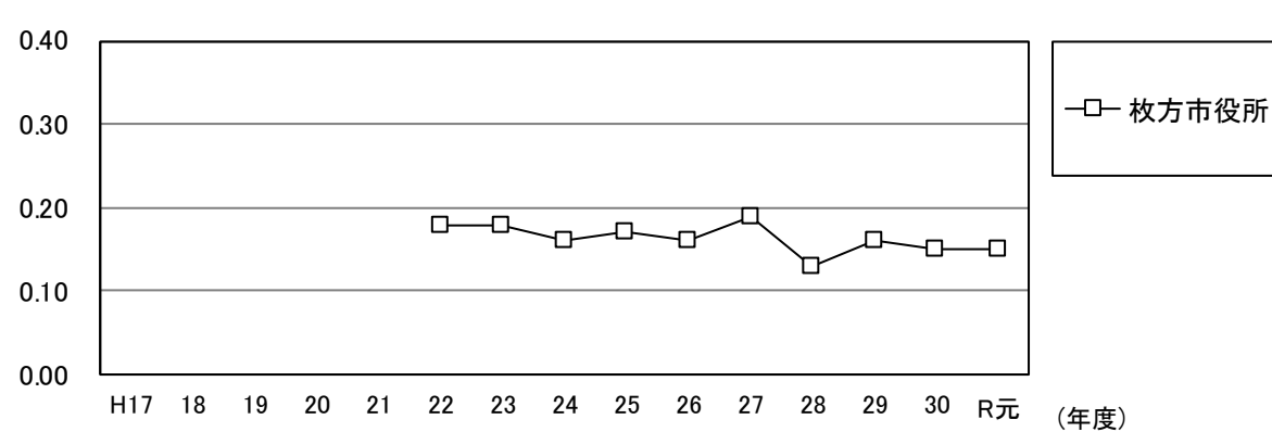
図 1-20 非メタン炭化水素の午前6～9時における年平均値の経年変化（一般局）
