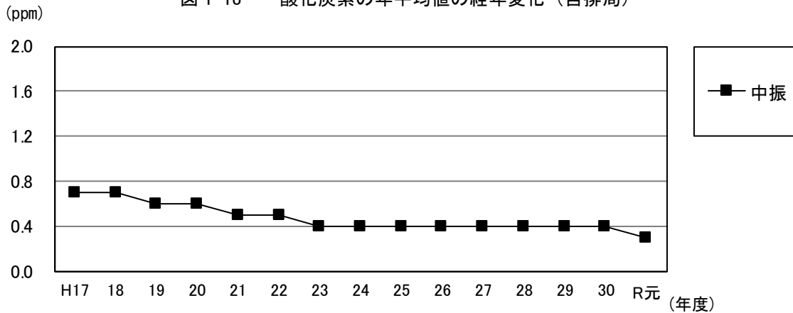
図 1-18 一酸化炭素の年平均値の経年変化（自排局）
