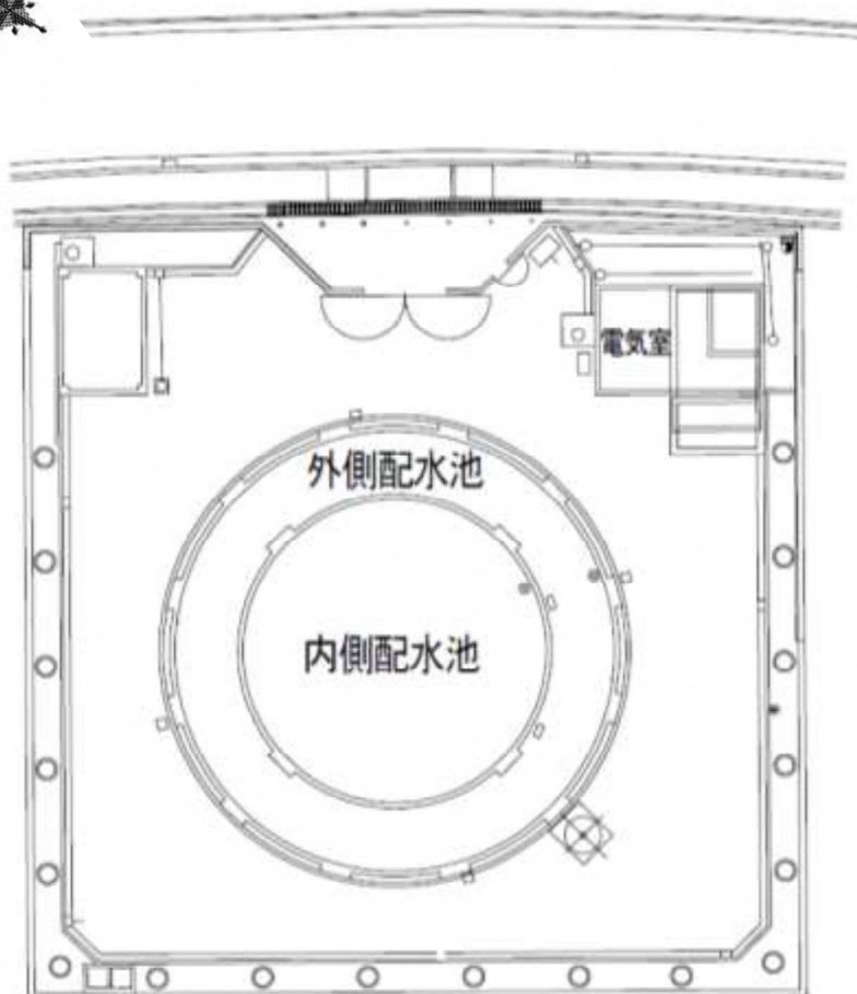
長尾宮前配水場平面図
