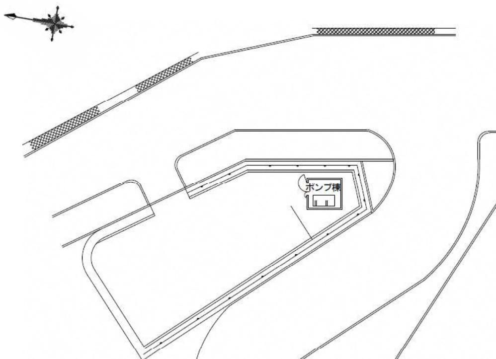
穂谷加圧ポンプ室平面図
