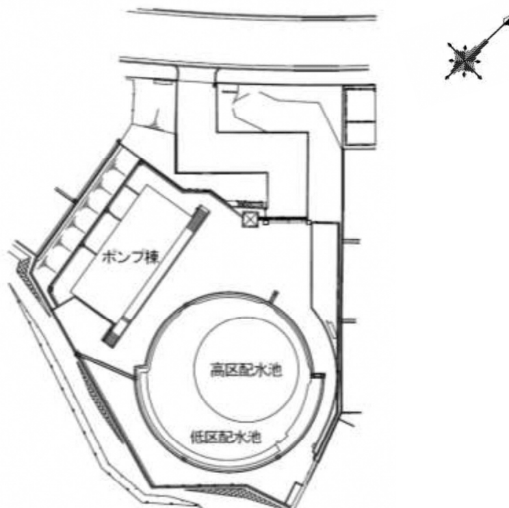
北山配水場平面図
