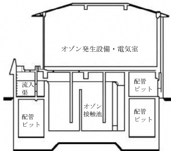
⑤ オゾン処理棟断面図
