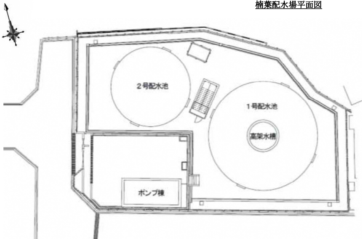
楠葉配水場平面図
