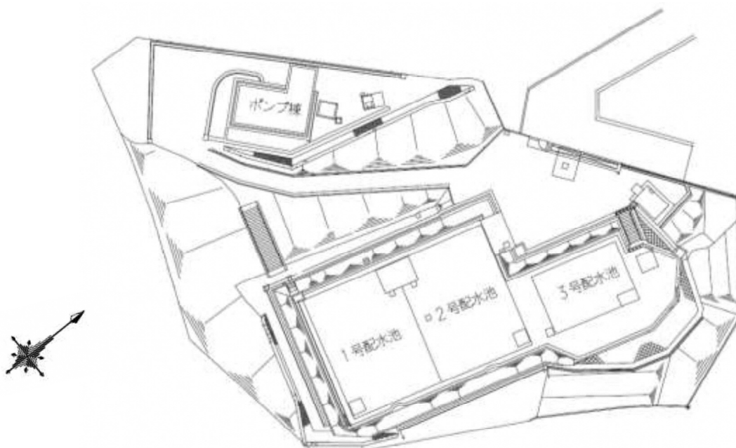
尊延寺配水場平面図
