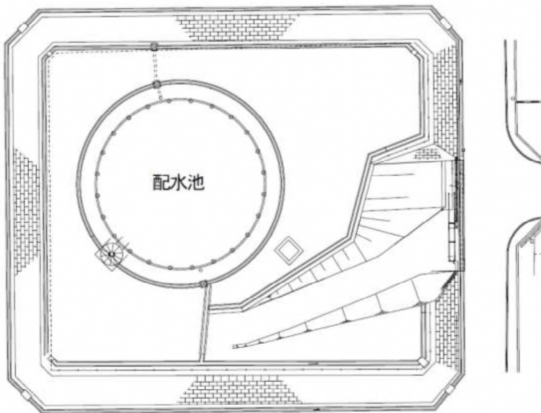
北部長尾配水池平面図
