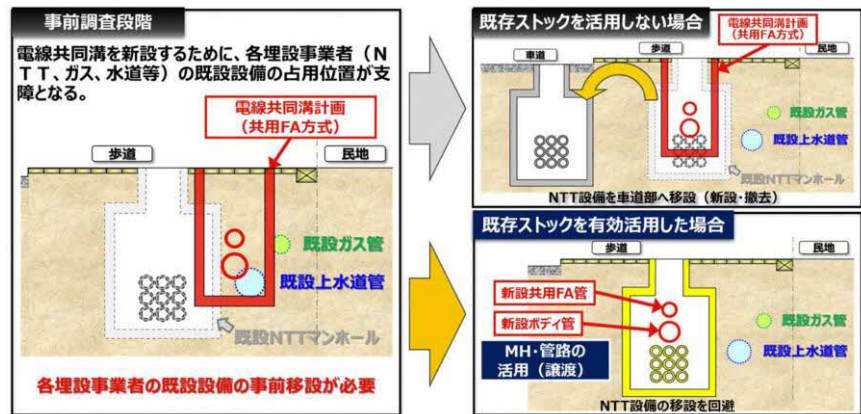
図 5-2 既存ストック活用（マンホール）のイメージ
