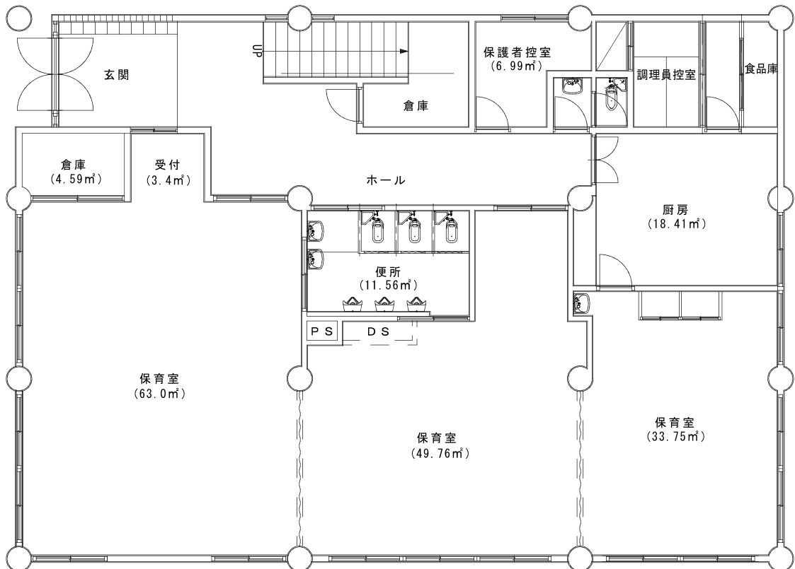
1 F 平面図 S=1/100
