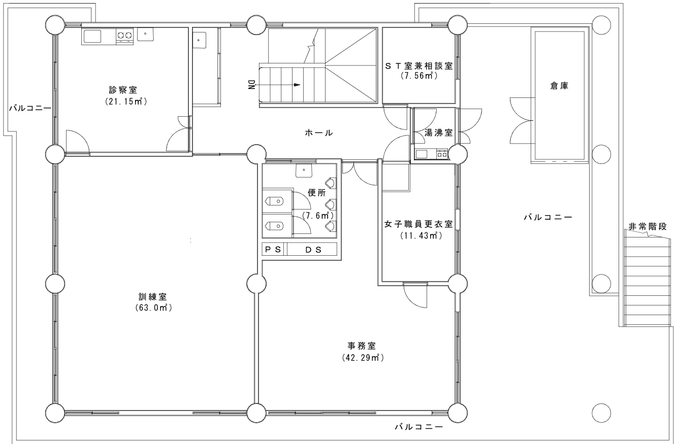
2 F 平面図 S=1/100
