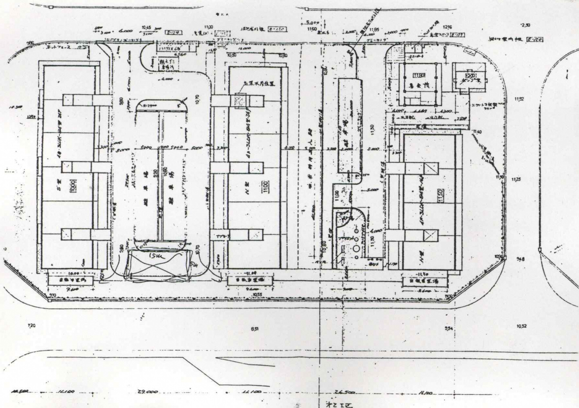
配置図
