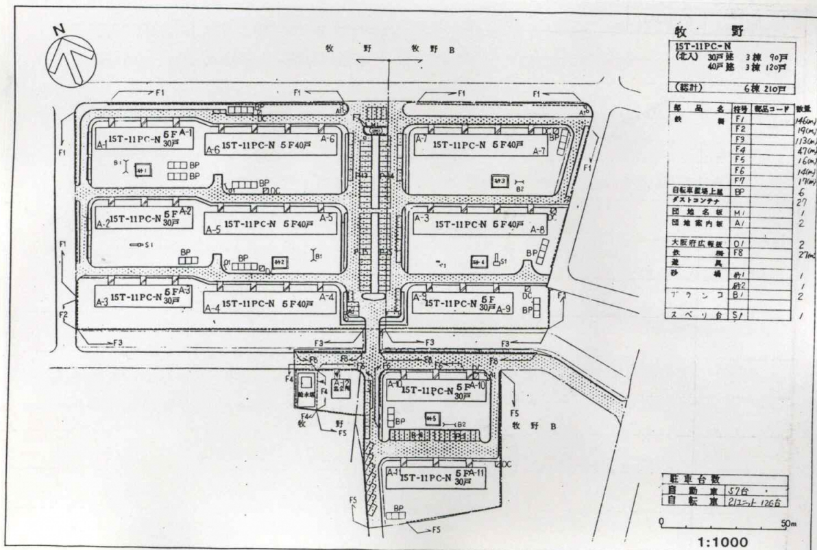
配置図
