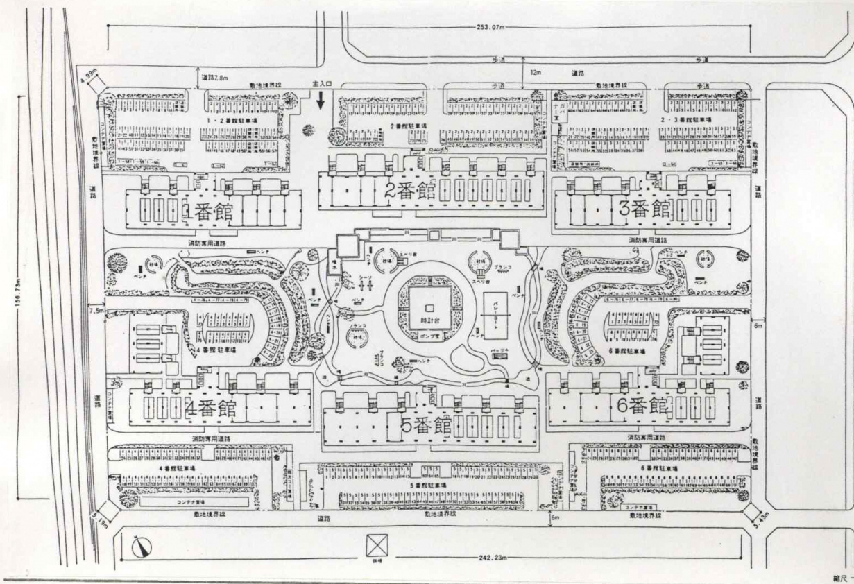
配置図
