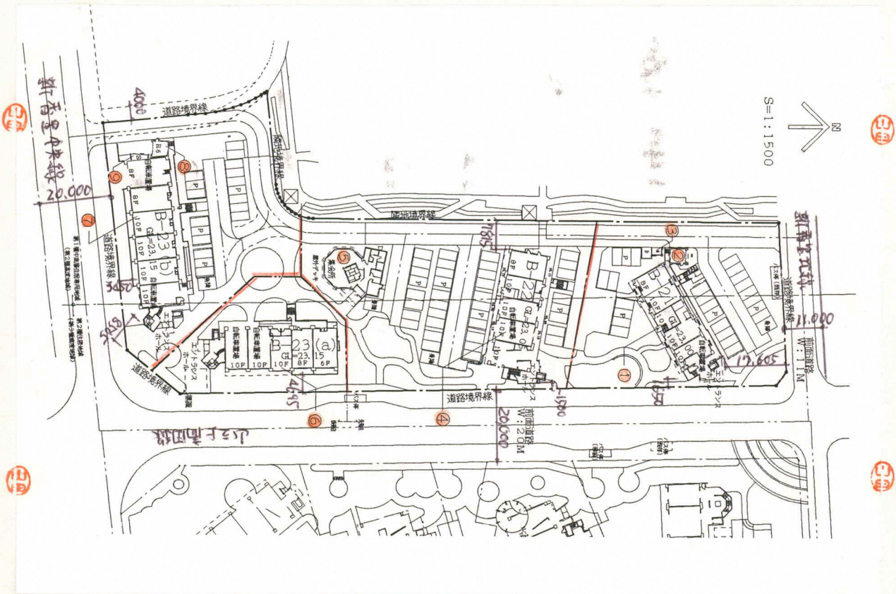
配置図
