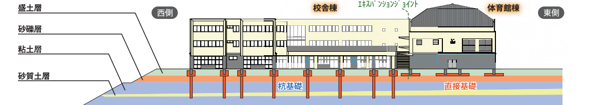
【図3-7 想定される地盤と基礎形式の考え方の概念図】
