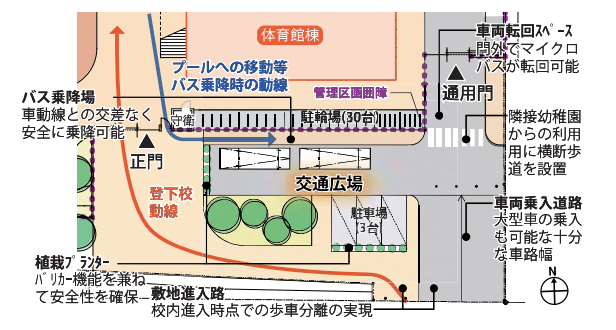
【図1-5 交通広場説明図】
