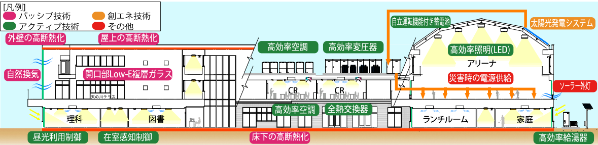
【図3-6 ZEB Ready達成のための導入設備概念図】
