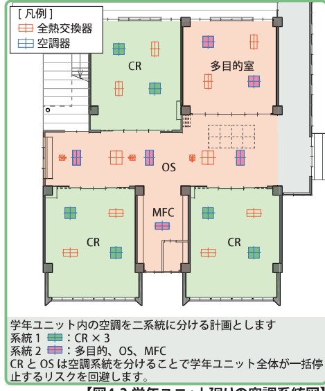
【図4-3 学年ユニット廻りの空調系統図】
