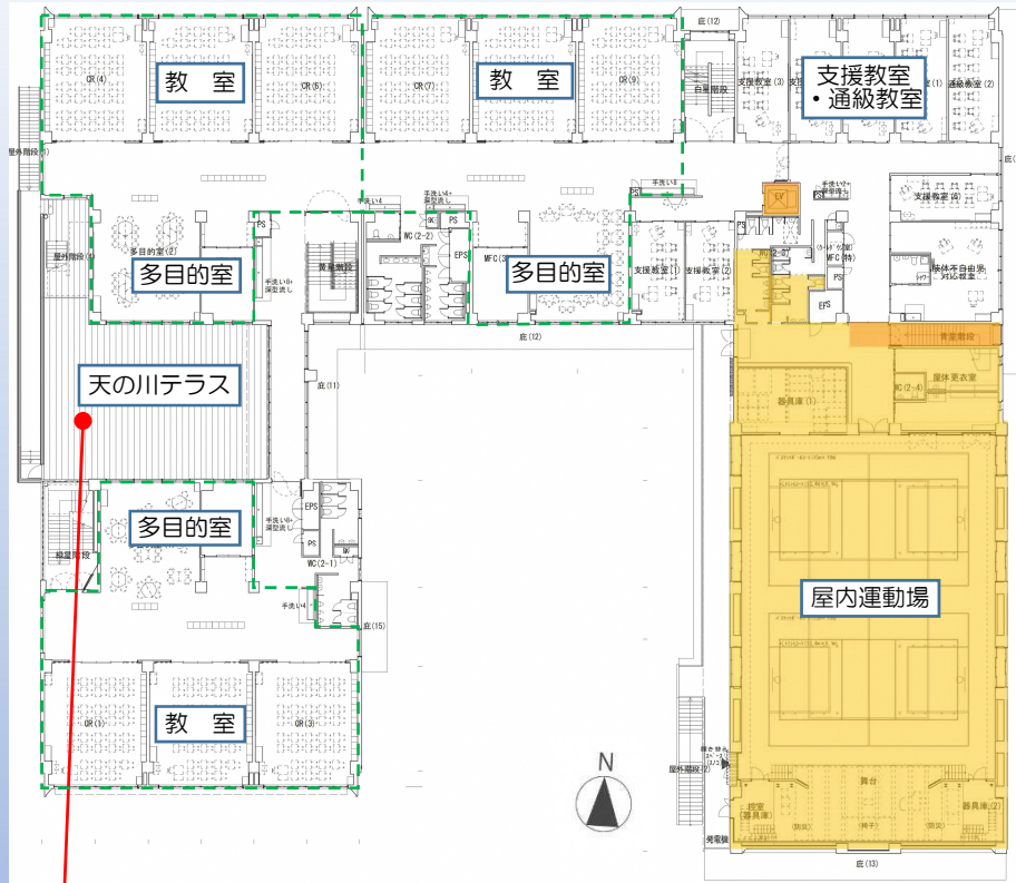
2階平面図
