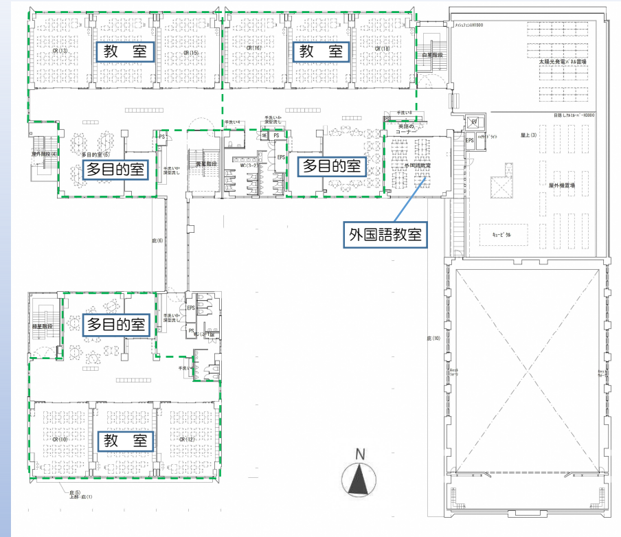
3階平面図
