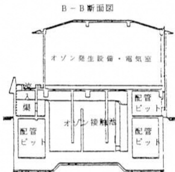
⑤ オゾン処理棟断面図
