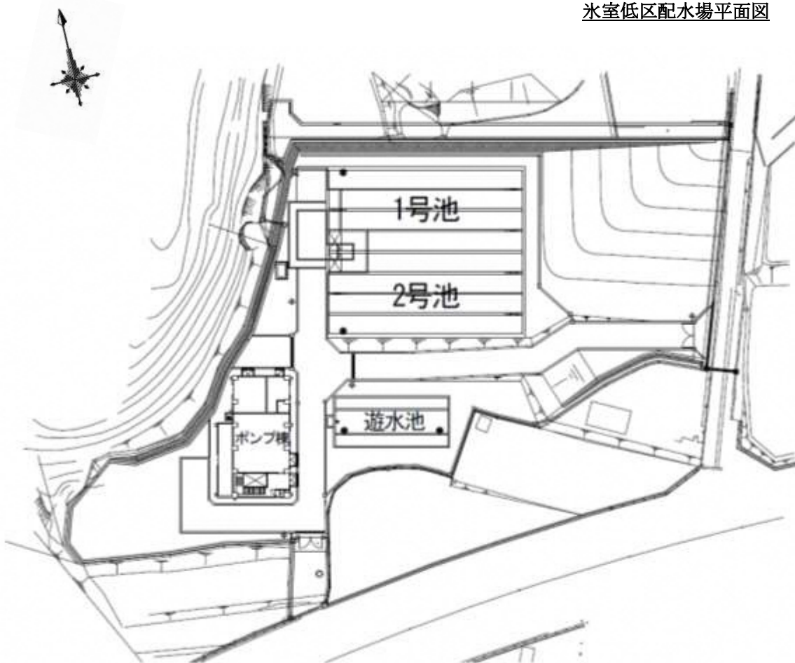
氷室低区配水場平面図
