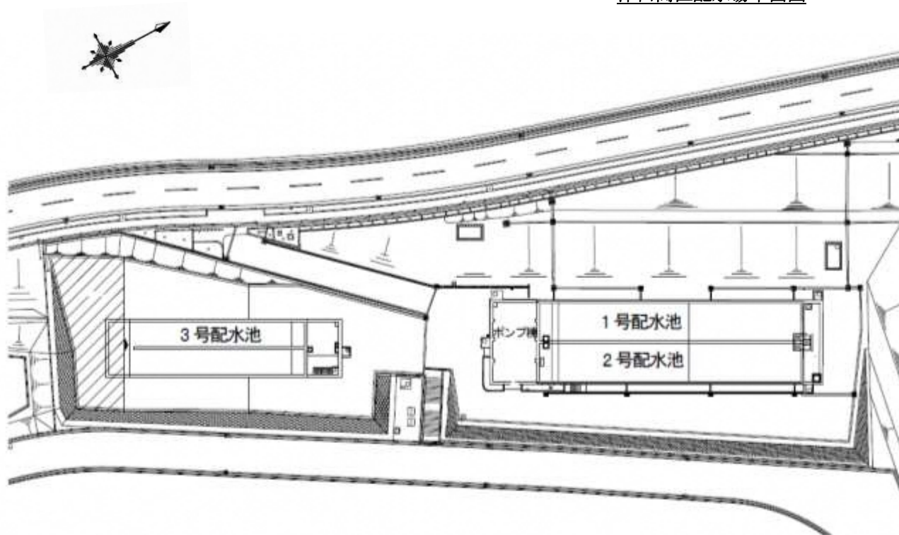
津田高区配水場平面図
