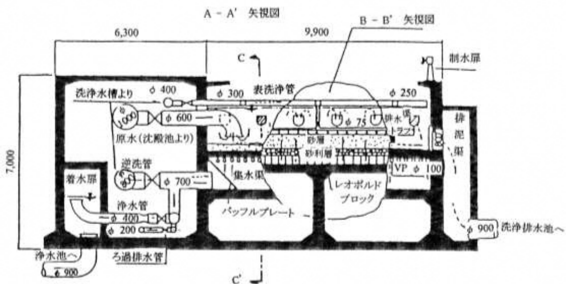
④ 急速ろ過池断面図
