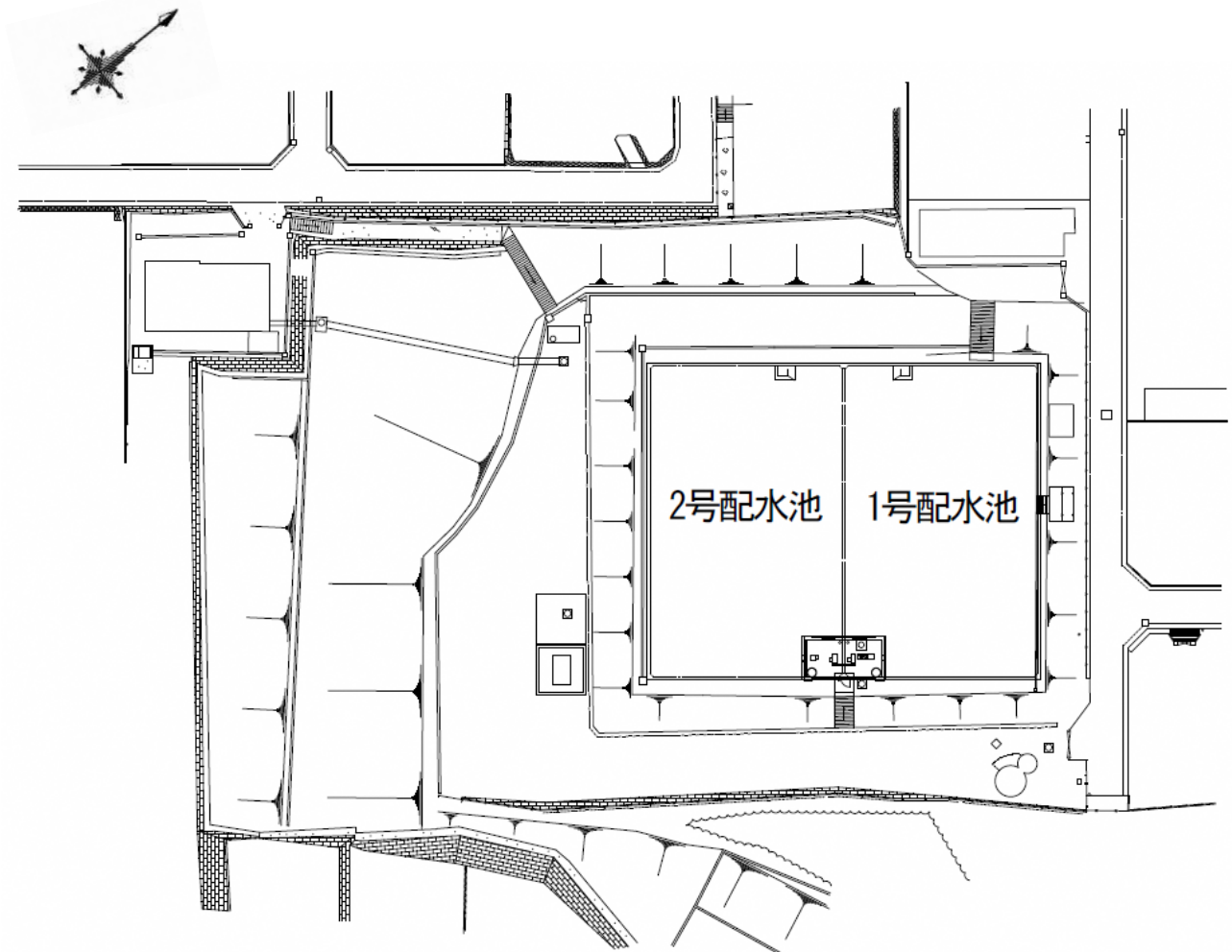
東部長尾配水場平面図
