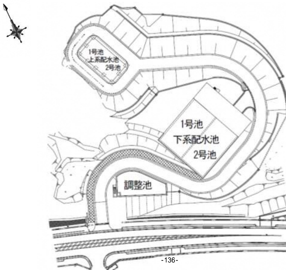
氷室高区配水場平面図
