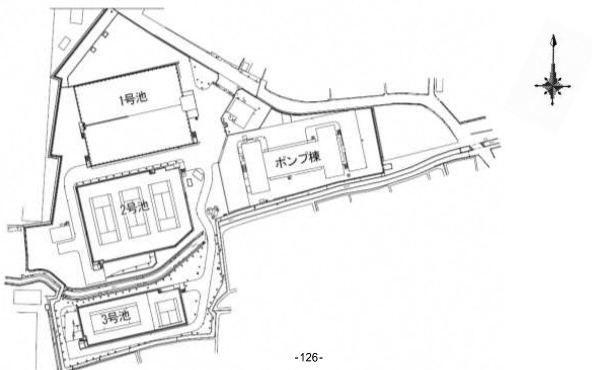
春日受水場平面図
