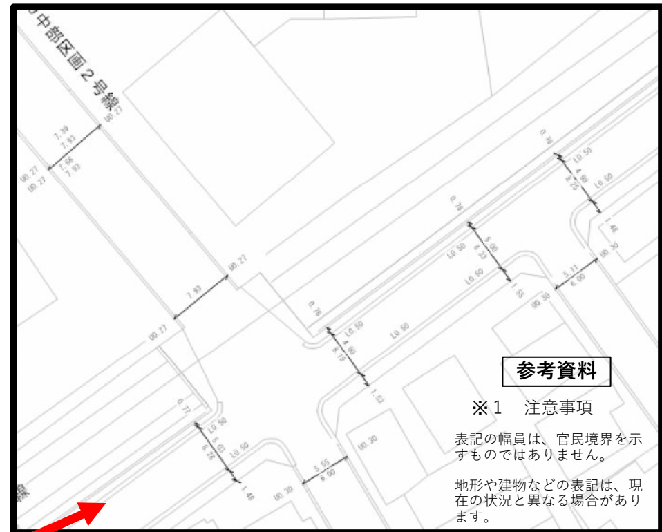
公開図面（道路台帳現況平面図）
