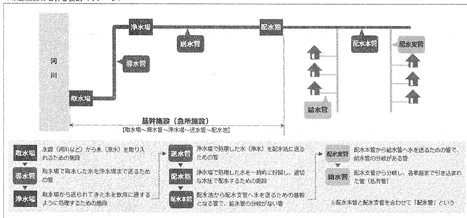
▼水道施設の名称と役割（イメージ）
