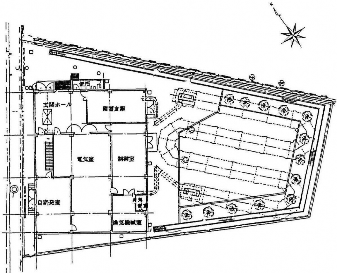
香里受水場平面図
