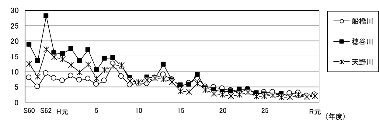
図 2-3 環境基準点でのBODの年平均値の経年変化
