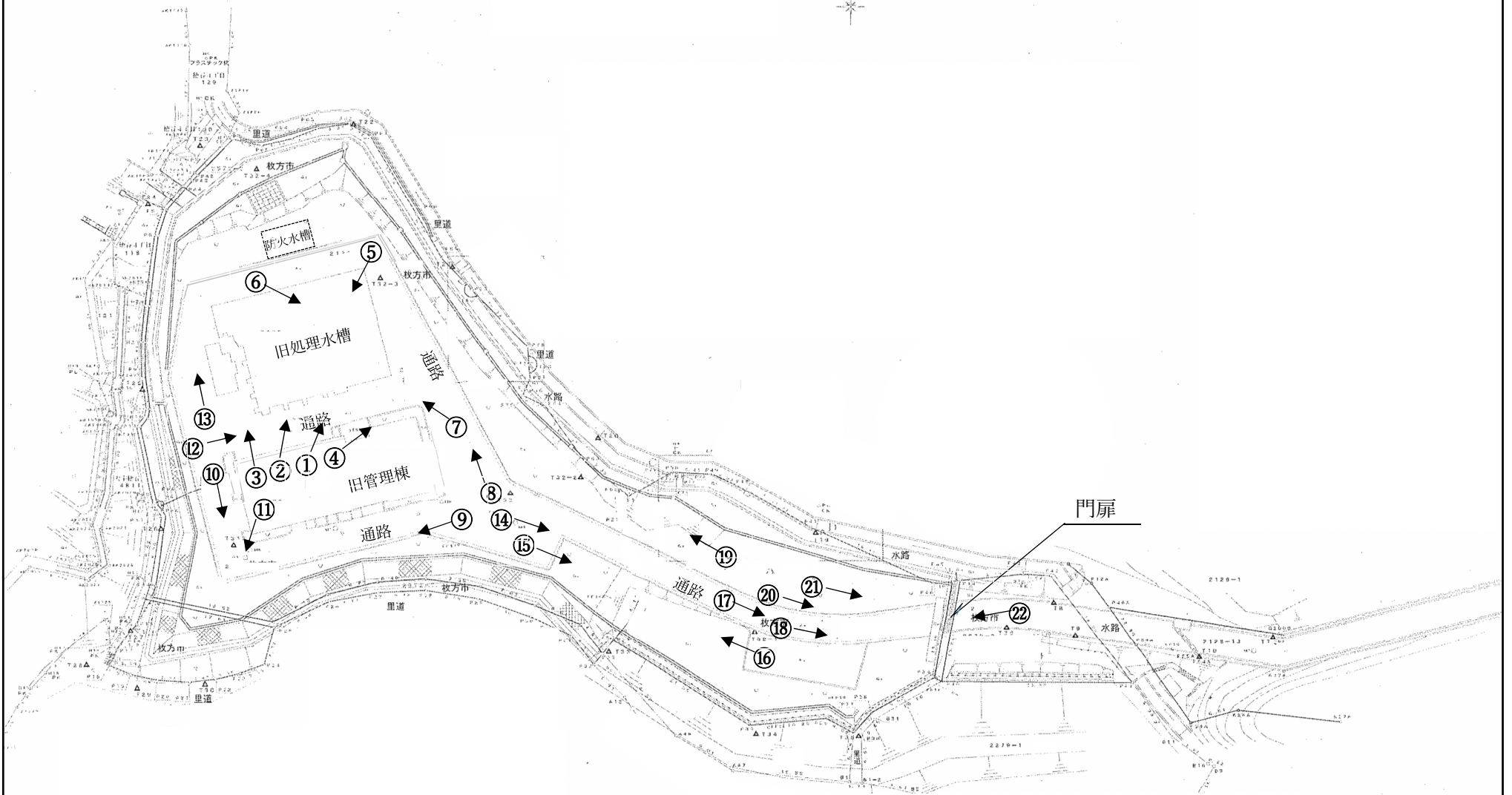
枚方市一般廃棄物最終処分場排水処理施設 平面図
