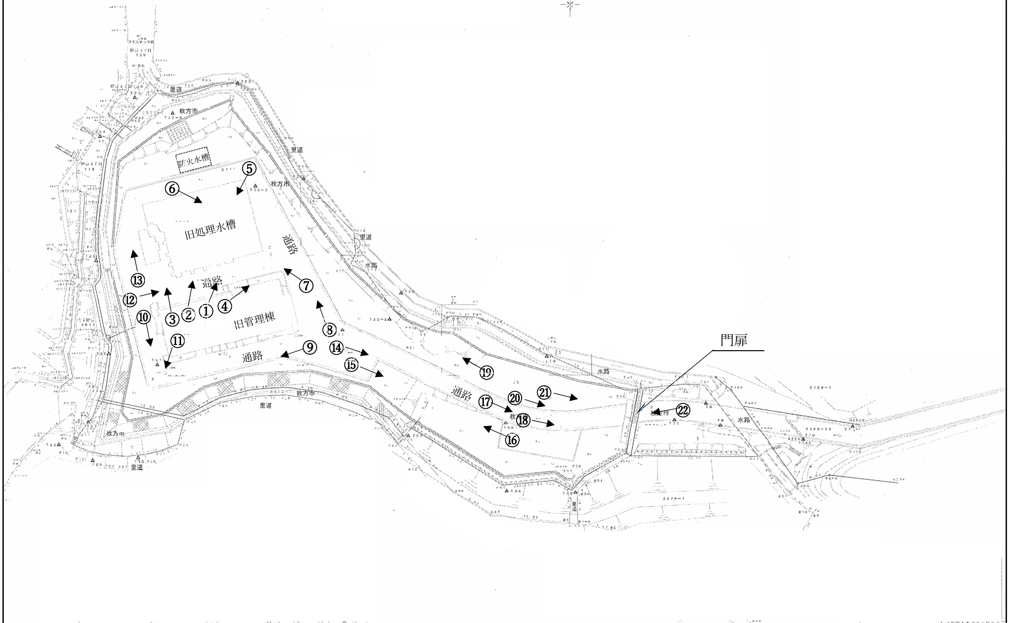
枚方市一般廃棄物最終処分場排水処理施設 平面図
