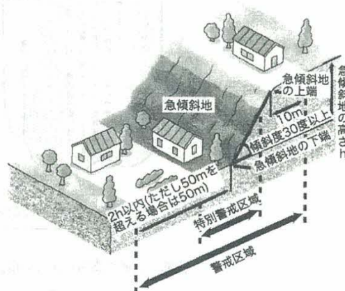
急傾斜地の崩壊に係る土砂災害警戒区域等の模式図
