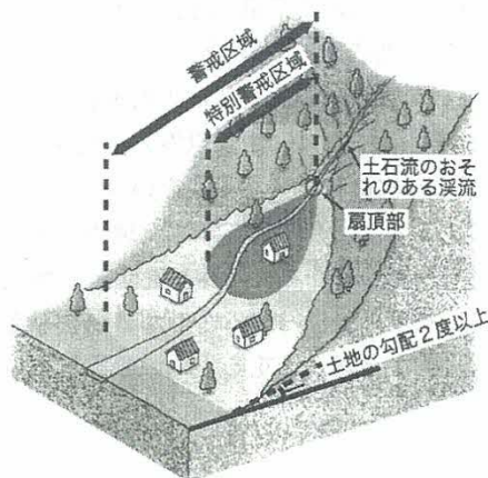
土石流に係る土砂災害警戒区域等の模式図
