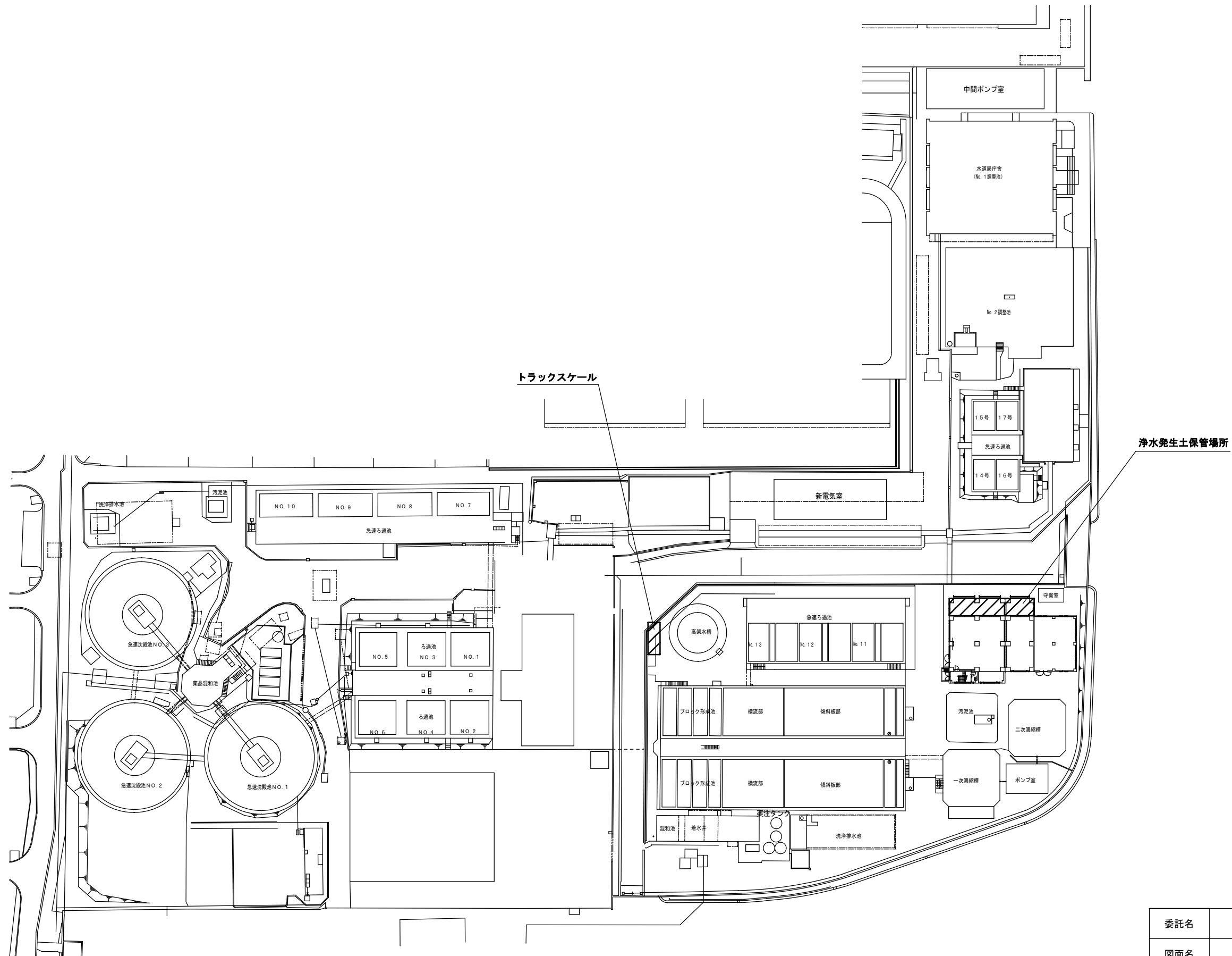
全体平面図
