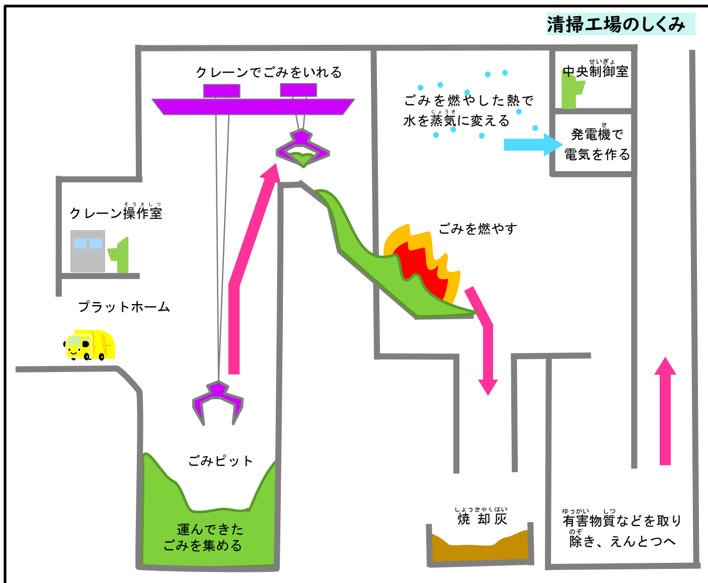
↑ 枚方市の燃えるゴミを処理するしくみ
