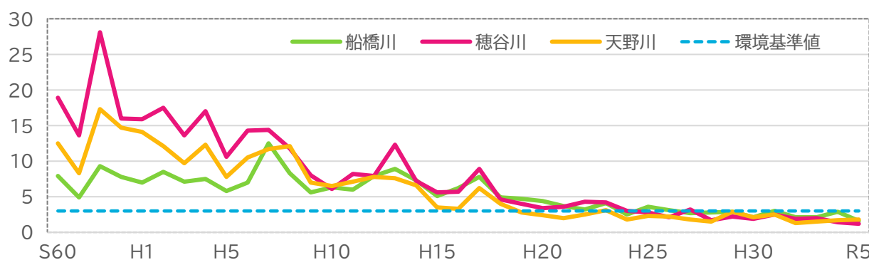
↑ 枚方市の主な川のよごれの変化 川のよごれの目安としてBOD（生物化学的酸素要求量）の移り変わりをグラフにしています。
