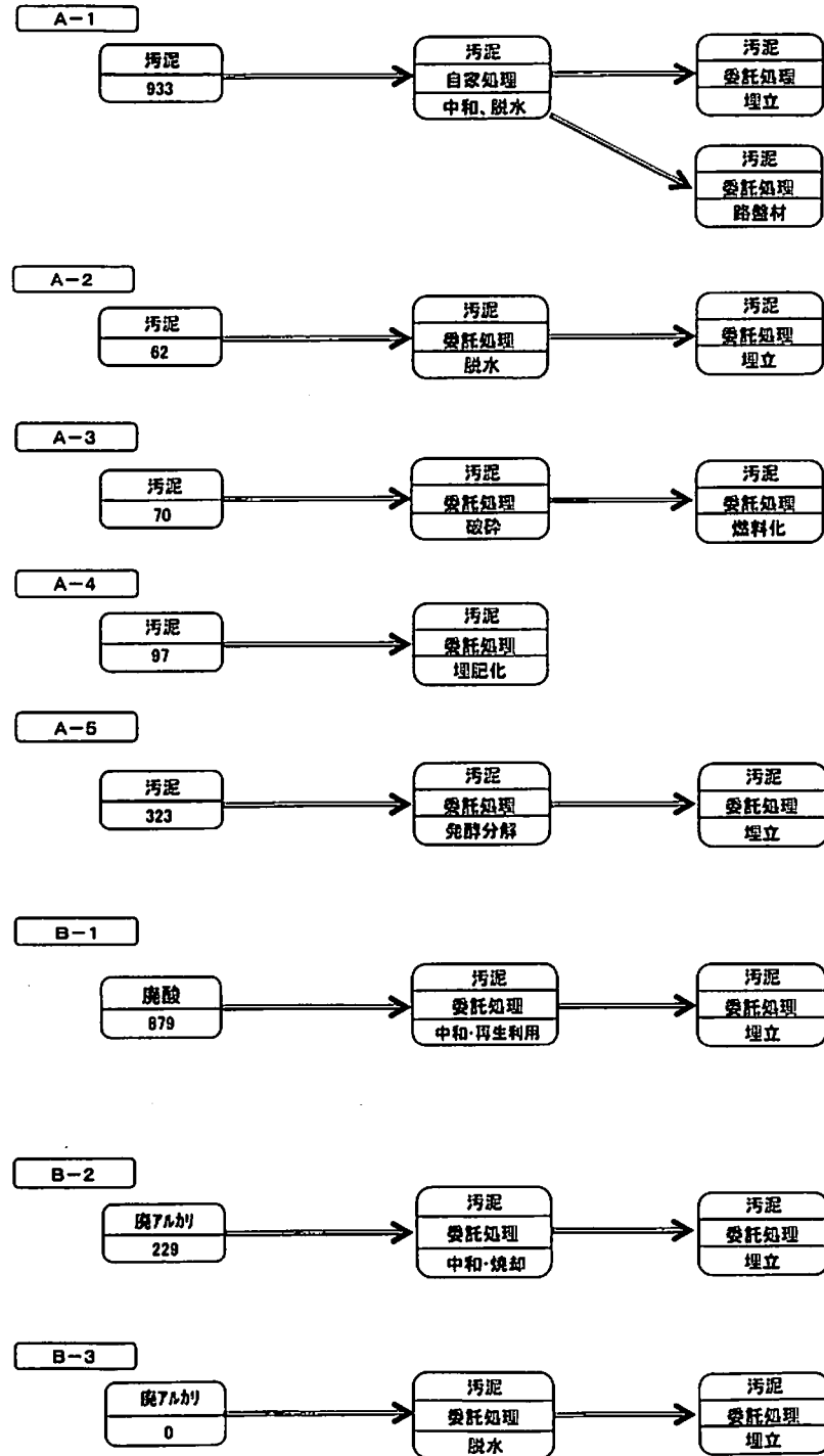
2015年度産業廃棄物処理工程フロー図
