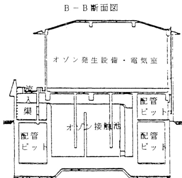
⑤ オゾン処理棟断面図
