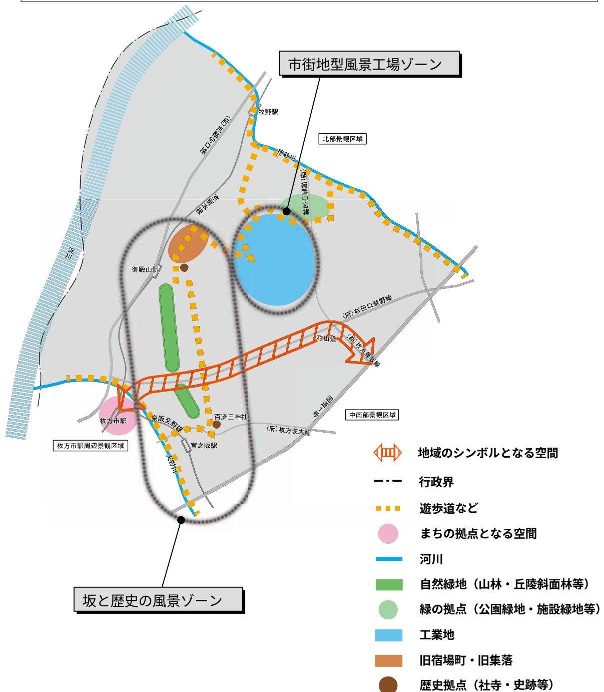
中部景観区域 景観形成概念図
