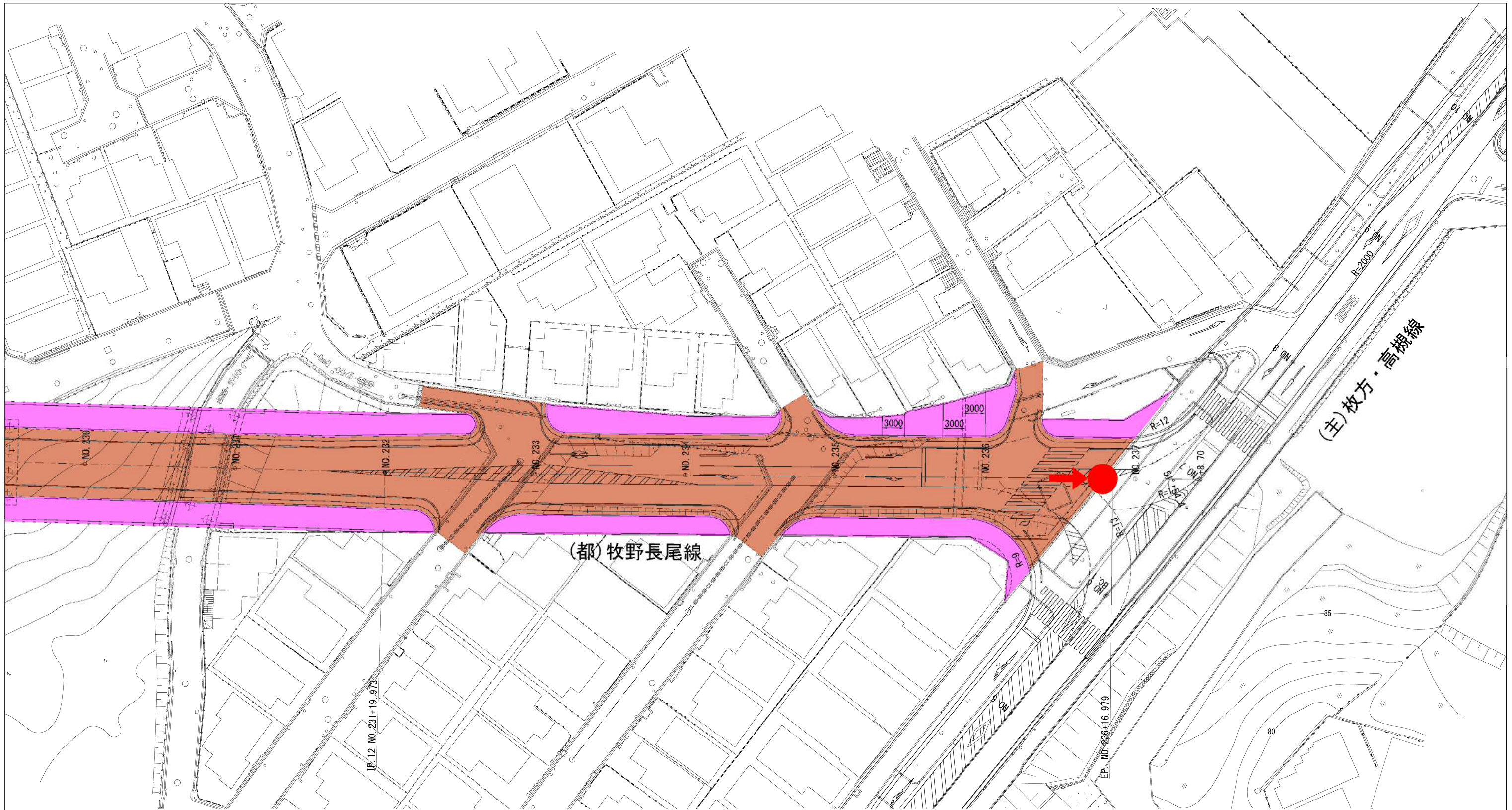
府道枚方高槻線付近断面図
