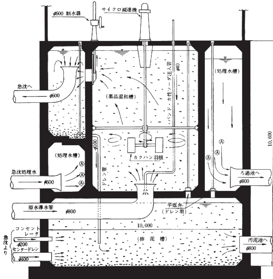
① 薬品混和池断面図 (八角槽)
