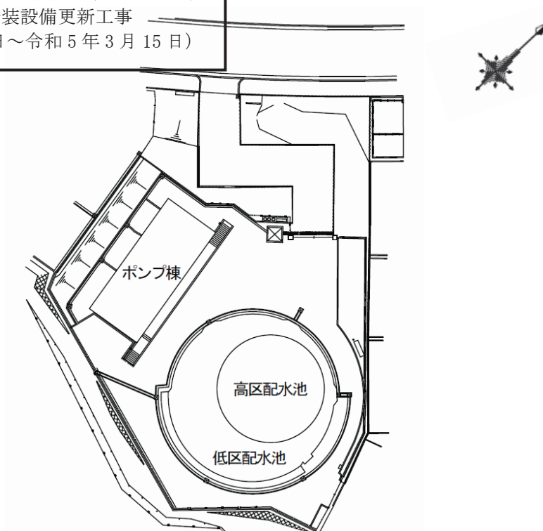
北山配水場平面図
