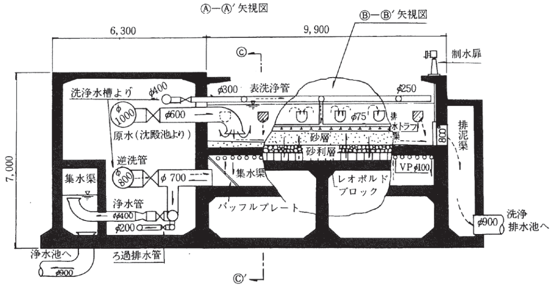
④ 急速ろ過池断面図
