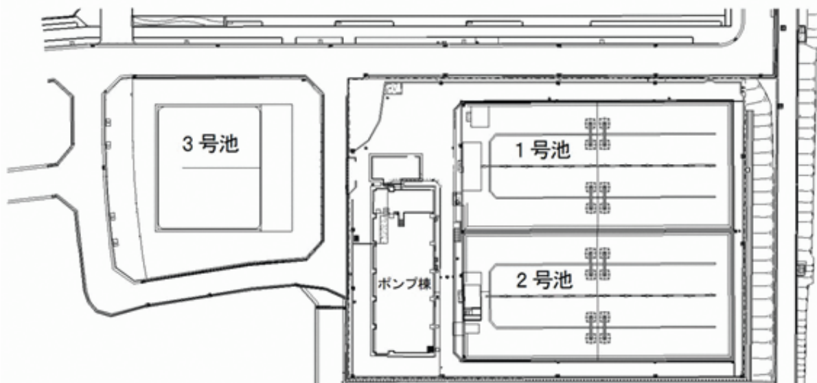
田低区配水場平面図
