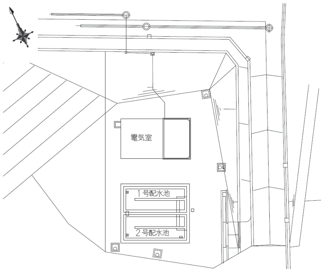
国見山配水池平面図
