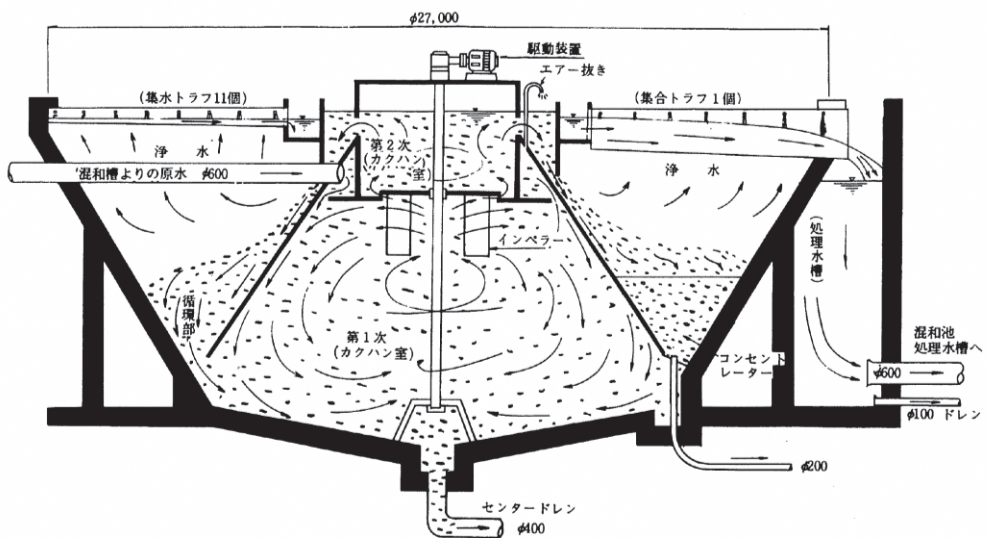
② 急速沈殿池断面図
