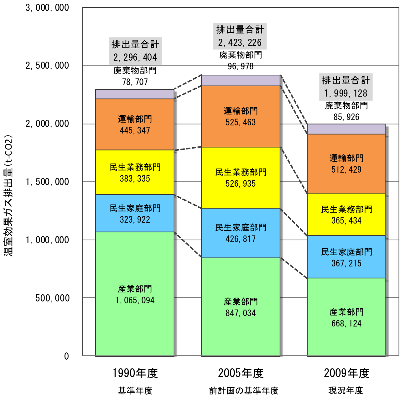
図 部門別温室効果ガス排出量の動向
