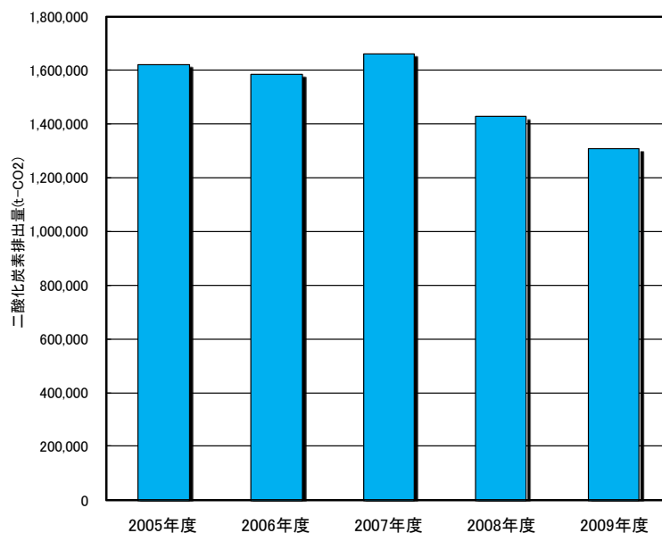
図 前計画の算定方法による市域の二酸化炭素排出量の推移 1
