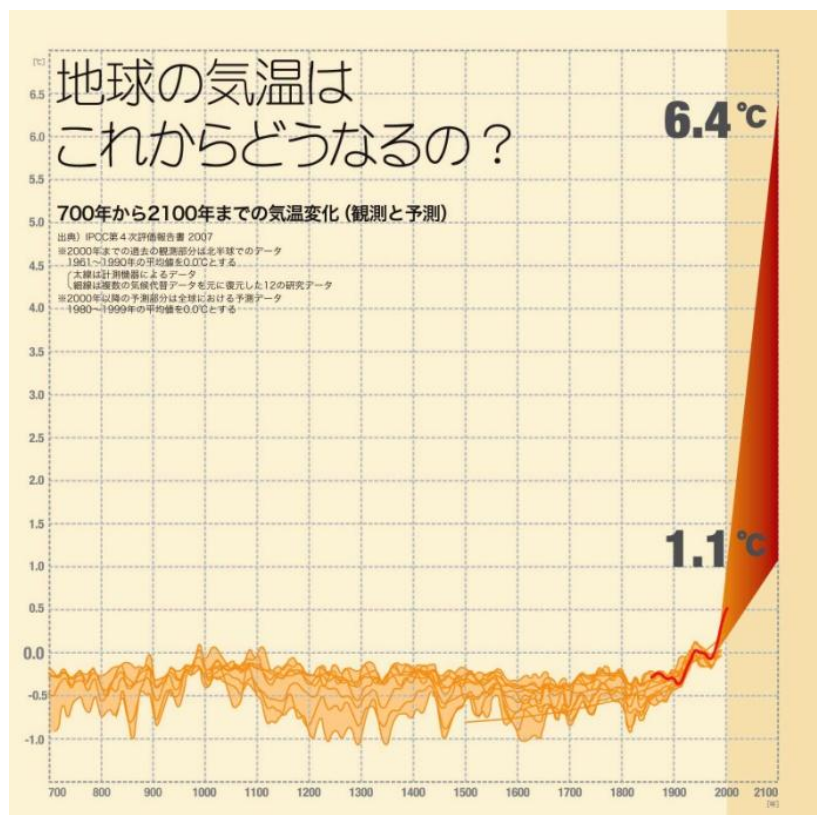
図 気温変動（観測と予測）
