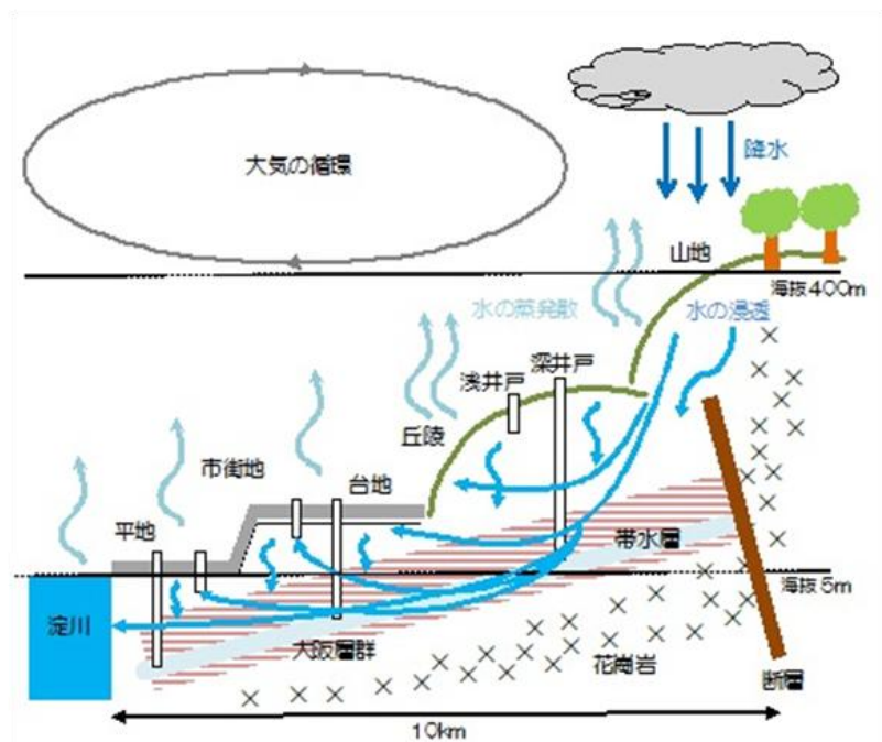
図 地形地質断面の概念図
