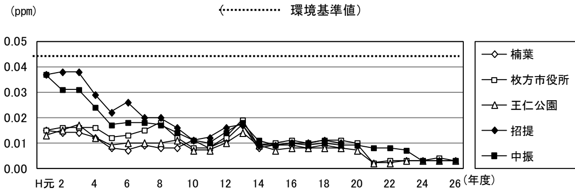
図 1-4 二酸化硫黄の年間 2%除外値の推移と環境基準値との比較
