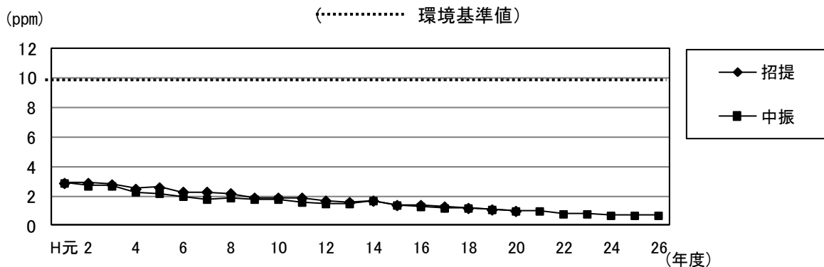
図 1-5 一酸化炭素の年間 2%除外値の推移と環境基準値との比較
