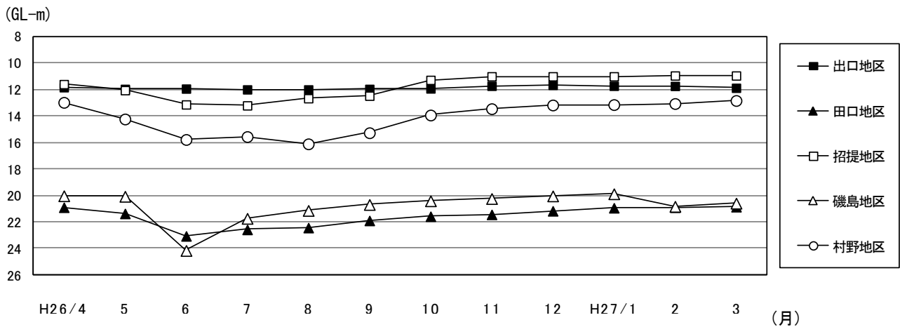
図 4-2 地下水位（静水位）の月平均値の変化
