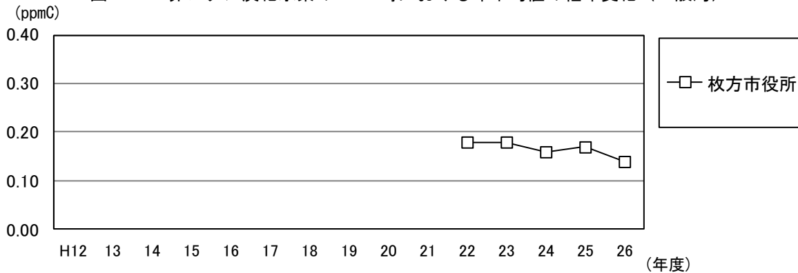
図 1-20 非メタン炭化水素の6～9時における年平均値の経年変化（一般局）
