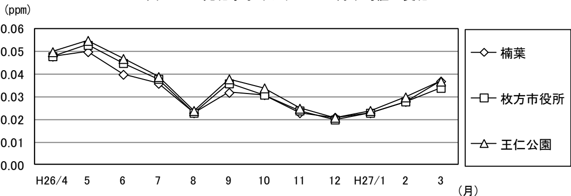
図 1-15 光化学オキシダントの月平均値の変化
