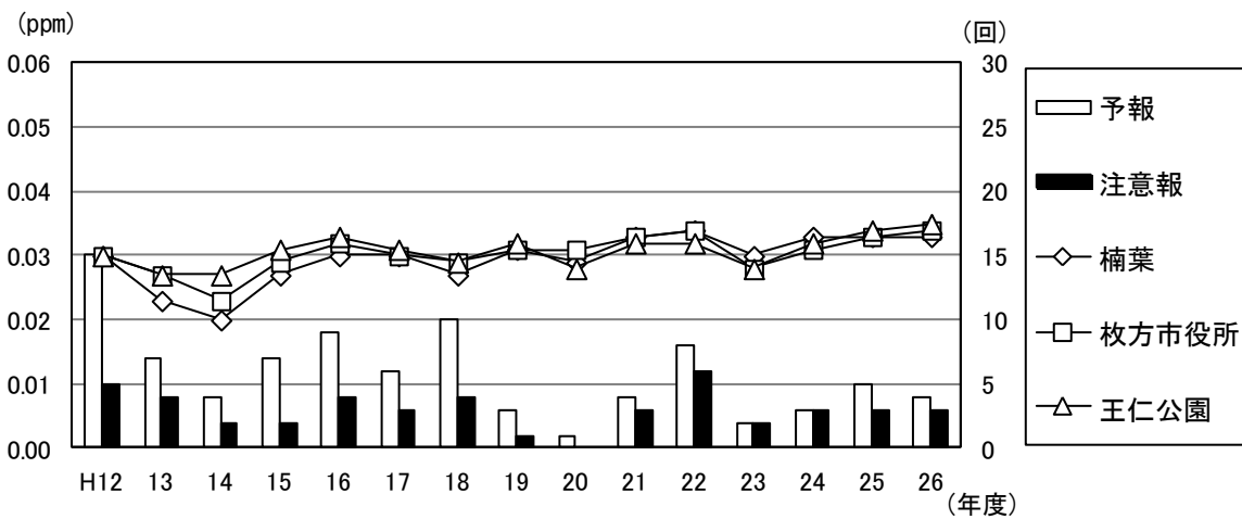
図 1-14 光化学オキシダントの昼間1時間値の年平均値の経年変化と光化学スモッグ発令回数の推移
