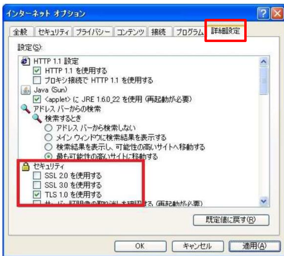
図. Internet Explorer 6 の設定
